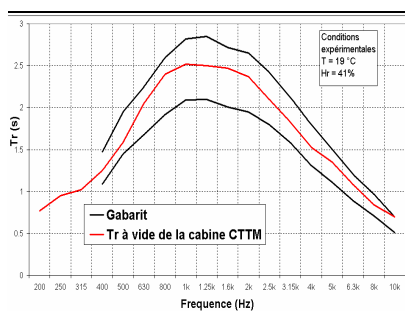
Temps de réverbération à vide et gabarit D49-1998
