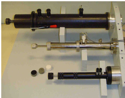
Tubes de Kundt CTTM : diamètres 29, 45 et 100 mm
